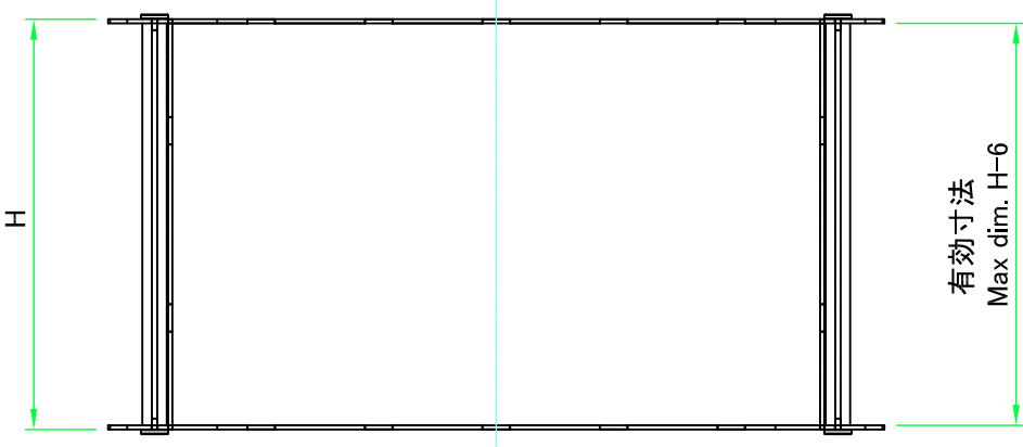
Wパネル1 / W panel 1
