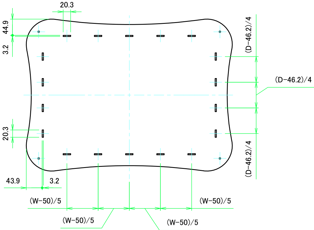
上カバー裏面 / Top cover Backside
